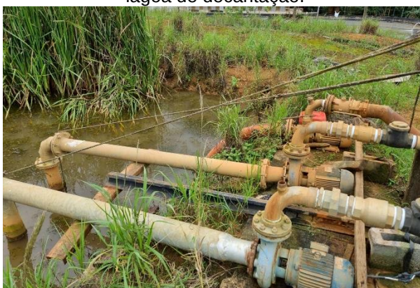
Figura 19: Sistema de recirculação de água na lagoa de decantação.
